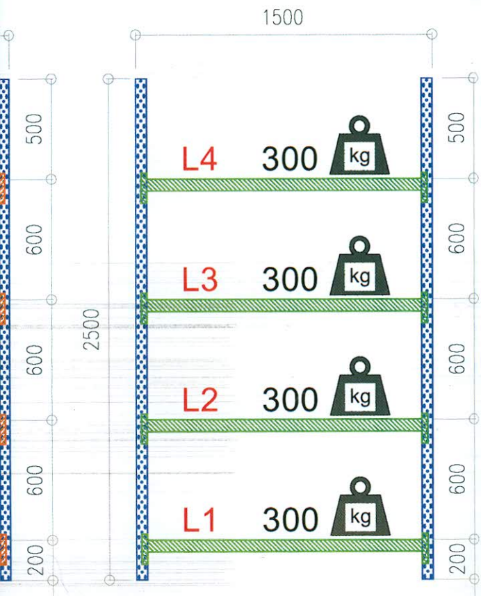
ELEVATION 1:25
